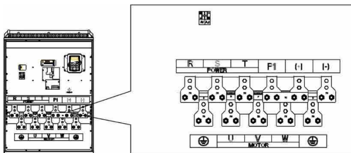
Fig 4-16 220~315kW
